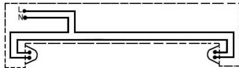
Schaltplan Lampengehäuse
